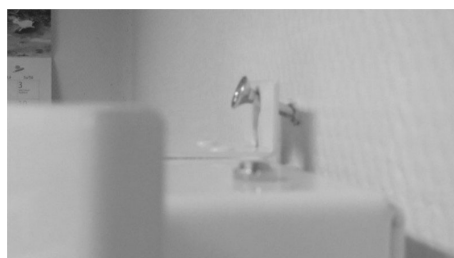
Fästsruven installeras lite snett uppåt, skruvhuvudet ca. 20 mm från väggen
